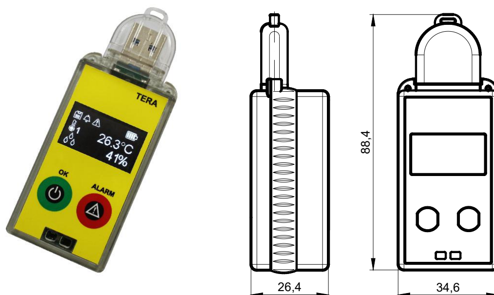
Рисунок 1 – Зовнішній вигляд логера
